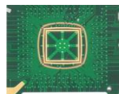
打線封裝載板
